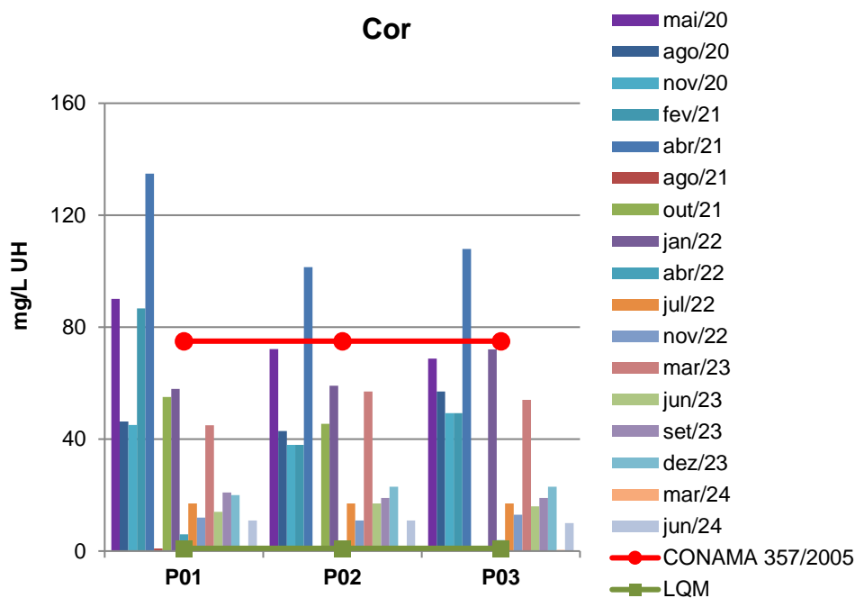
Figura 6 - Gráfico comparativo entre os resultados obtidos para Cor. Com o valor máximo estabelecido de 75 mg/L segundo a Resolução CONAMA 357/2005 e o valor do LQM (Limite de Quantificação do Método) para os pontos monitorados no rio Indaiá Grande- CGH Córrego.
