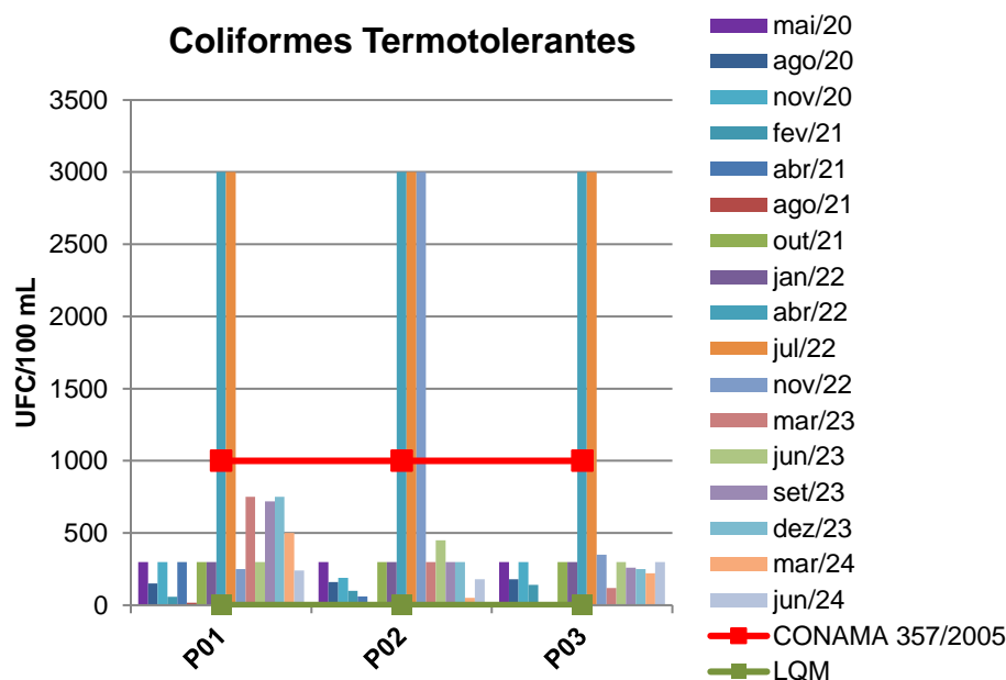
Figura 15 - Gráfico comparativo entre os resultados obtidos para Coliformes Termotolerantes, o valor máximo permitido segundo a Resolução CONAMA 357/2005) para os pontos monitorados no rio Indaiá Grande- CGH Córrego.
