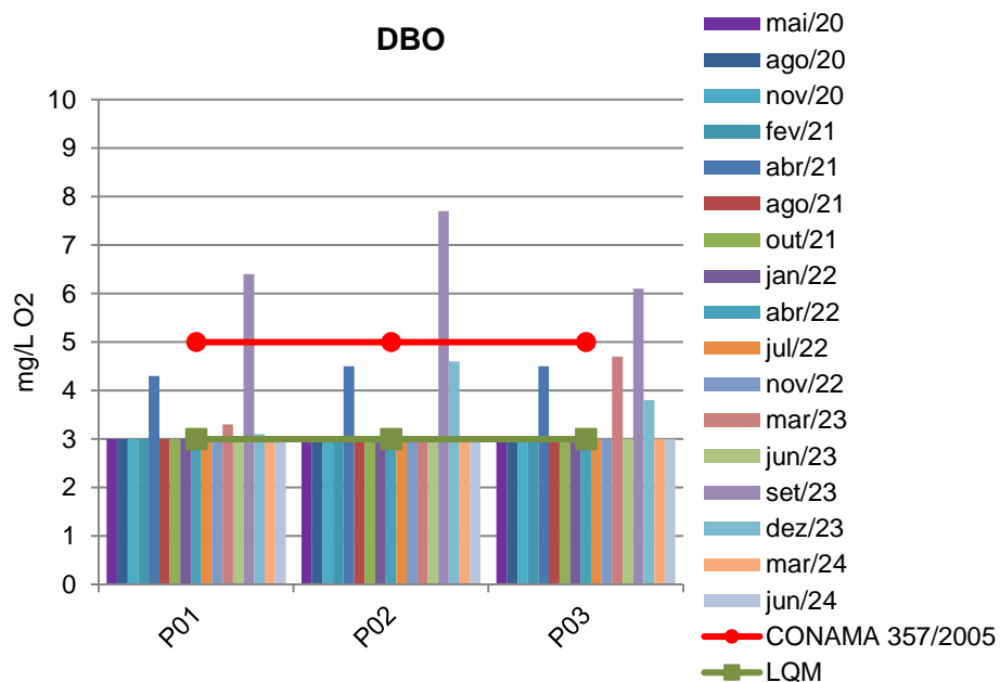
Figura 8 - Gráfico comparativo entre os resultados obtidos para DBO, o valor máximo permitido segundo a Resolução CONAMA 357/2005 e o LQM (Limite de Quantificação do Método) para os pontos monitorados no rio Indaiá Grande- CGH Córrego. ‘
