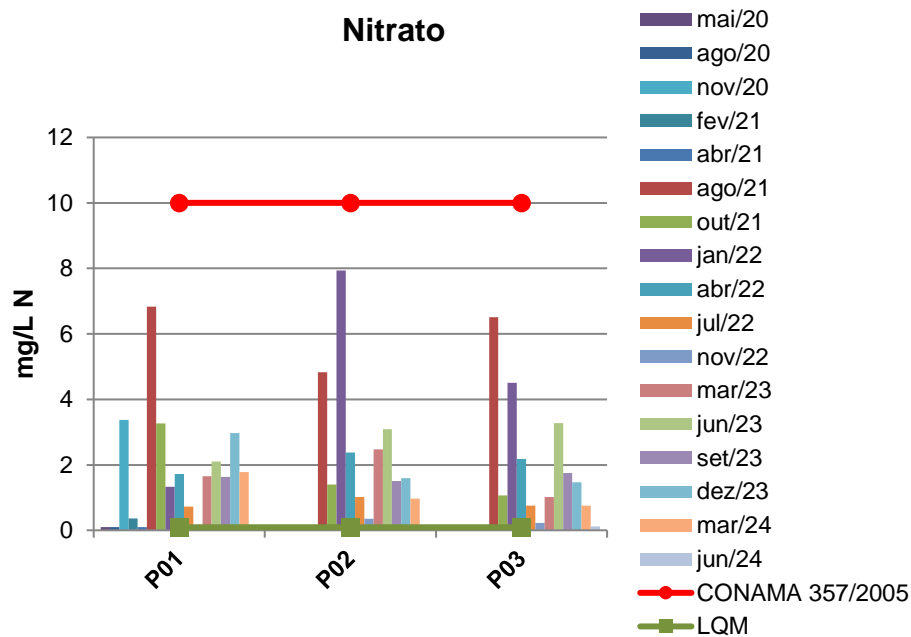
Figura 10 - Gráfico comparativo entre os resultados obtidos para Nitrito, o valor máximo permitido segundo a Resolução CONAMA 357/2005 e o LQM (Limite de Quantificação do Método) para os pontos monitorados no rio Indaiá Grande- CGH Córrego.
