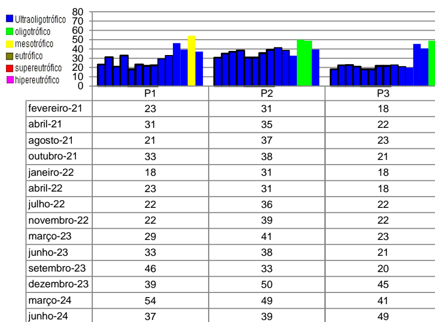
Figura 17 - Gráfico comparativo entre os resultados obtidos de IET para os pontos monitorados no rio Indaiá Grande- CGH Córrego.
