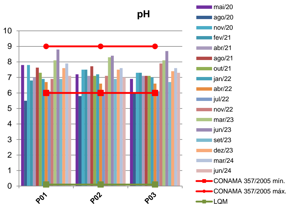
Figura 13 - Gráfico comparativo entre os resultados obtidos para pH, o valor máximo permitido segundo a Resolução CONAMA 357/2005 e o valor do LQM (Limite de Quantificação do Método) para os pontos monitorados no rio Indaiá Grande- CGH Córrego.
