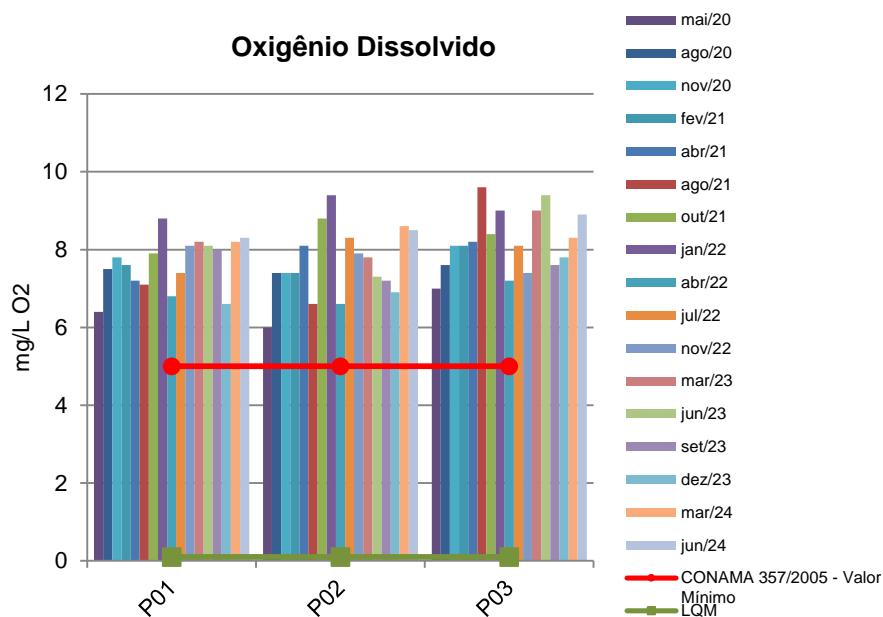
Figura 7 - Gráfico comparativo entre os resultados obtidos para Oxigênio Dissolvido, o valor mínimo permitido segundo a Resolução CONAMA 357/2005 e o valor do LQM (Limite de Quantificação do Método) para os pontos monitorados no rio Indaiá Grande- CGH Córrego.
