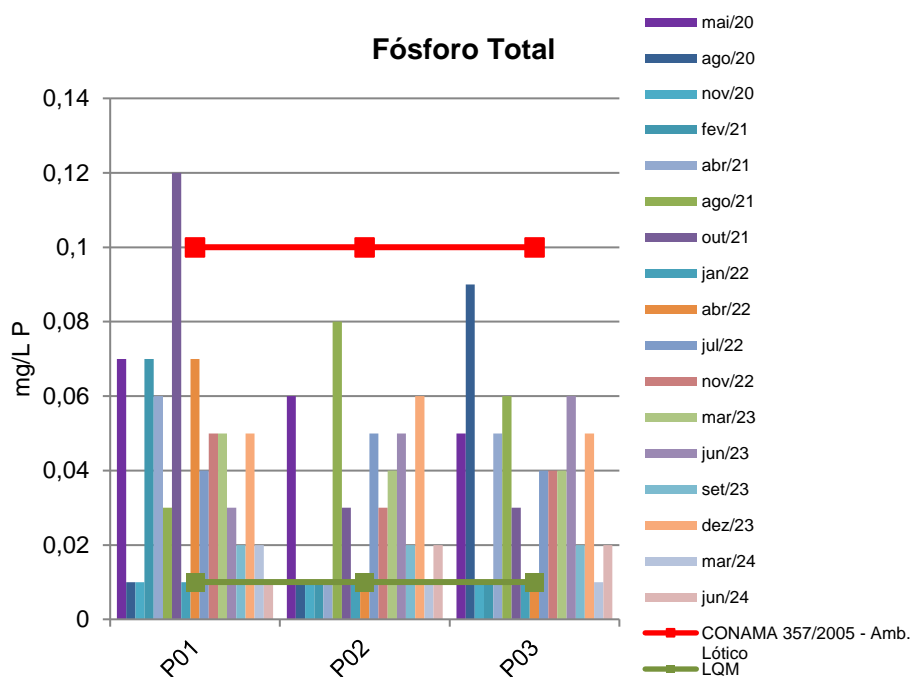
Figura 9 - Gráfico comparativo entre os resultados obtidos para Fósforo total, o valor máximo permitido segundo a Resolução CONAMA 357/2005 e o LQM (Limite de Quantificação do Método) para os pontos monitorados no rio Indaiá Grande- CGH Córrego.
