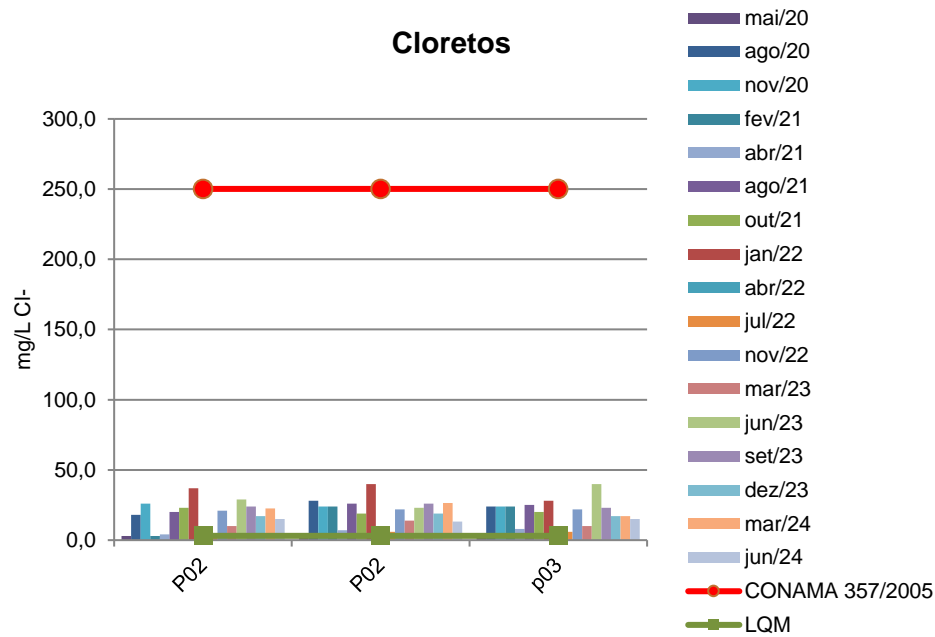
Figura 5 - Gráfico comparativo entre os resultados obtidos para Cloreto, o valor máximo permitido segundo a Resolução CONAMA 357/2005 e o valor do LQM (Limite de Quantificação do Método) para os pontos monitorados no rio Indaiá Grande- CGH Córrego.
