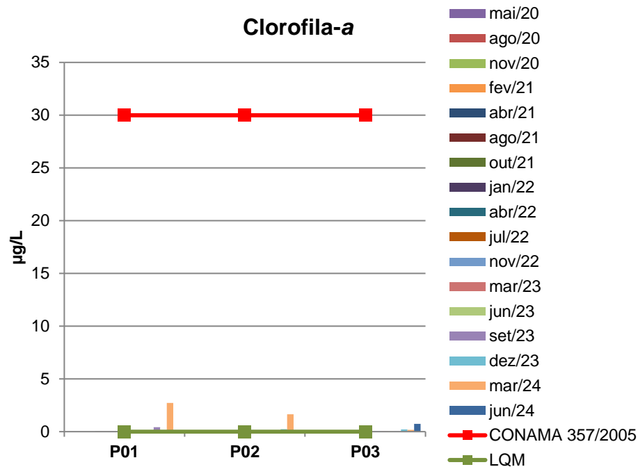
Figura 16 - Gráfico comparativo entre os resultados obtidos para Clorofila - a e o valor máximo permitido segundo a Resolução CONAMA 357/2005 para os pontos monitorados no rio Indaiá Grande- CGH. Todos os pontos apresentaram valores abaixo do limite de detecção do método.
